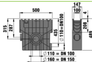
Ītekējimo dēzēs pjūvis
