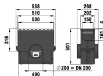
Ītekājimo dēzēs pjūvis
