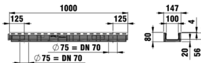
Latako pjūvis, tipas 80
