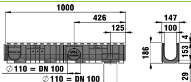
Latako pjūvis, tipas 010
