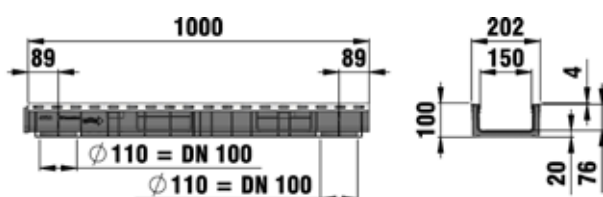
Latako pjūvis, tipas 100
