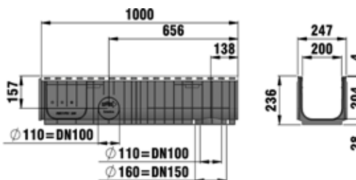
Latako pjūvis, tipas 020
