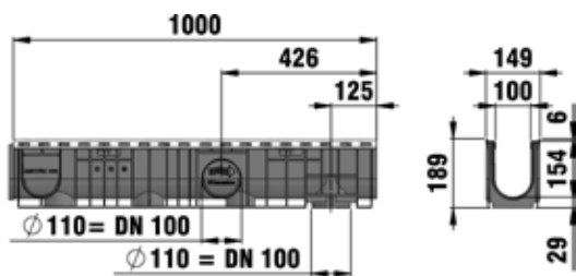
Latako pjūvis, tipas 010
