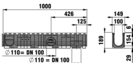
Latako pjūvis, tipas 010
