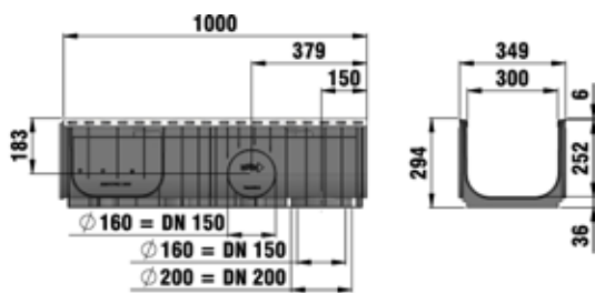
Latako pjūvis, tipas O1
