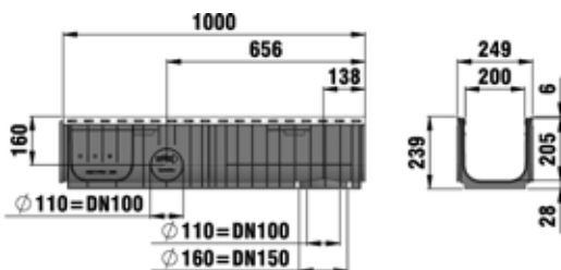
Latako pjūvis, tipas 020
