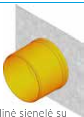
Galinė sienelė su horizontalia UPVC vamzdžio jungtimi DN 200, cinkuoto plieno, tipas O1
