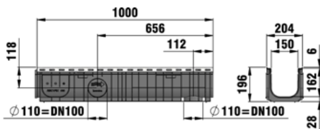
Latako pjūvis, tipas 01
