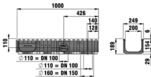
Latako pjūvis, tipas 010
