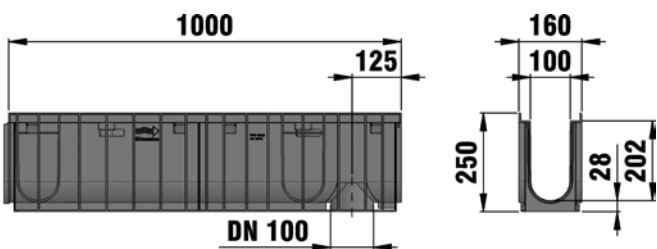
Latako pjūvis, tipas 020
