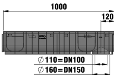
Latako pjūvis, tipas 01
