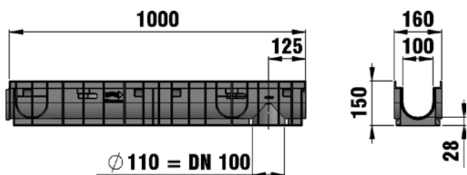
Latako pjūvis, tipas 01
