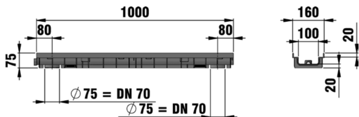
Latako pjūvis, tipas 75
