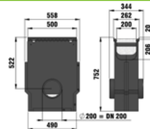
Įtekėjimo dėžės pjūvis
