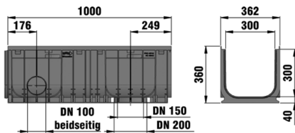
Latako pjūvis, tipas 010
