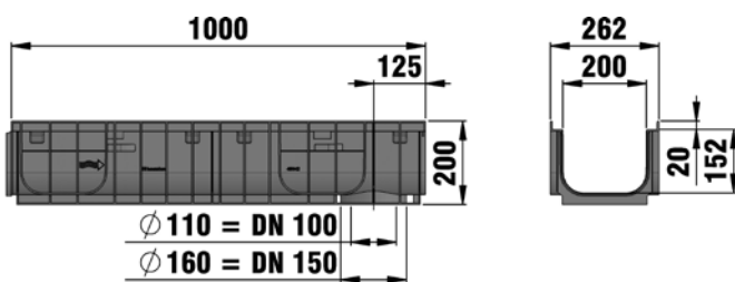
Latako pjūvis, tipas 010
