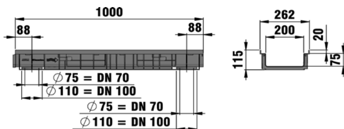
Latako pjūvis, tipas 115
