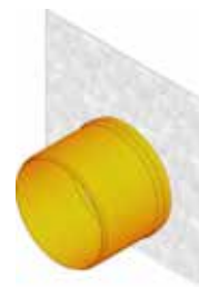
Galinē sienelē su vamzdžio jungtimi DN 200, tipas 010
